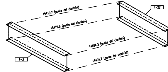
VISTA MISURE ESTERNE
