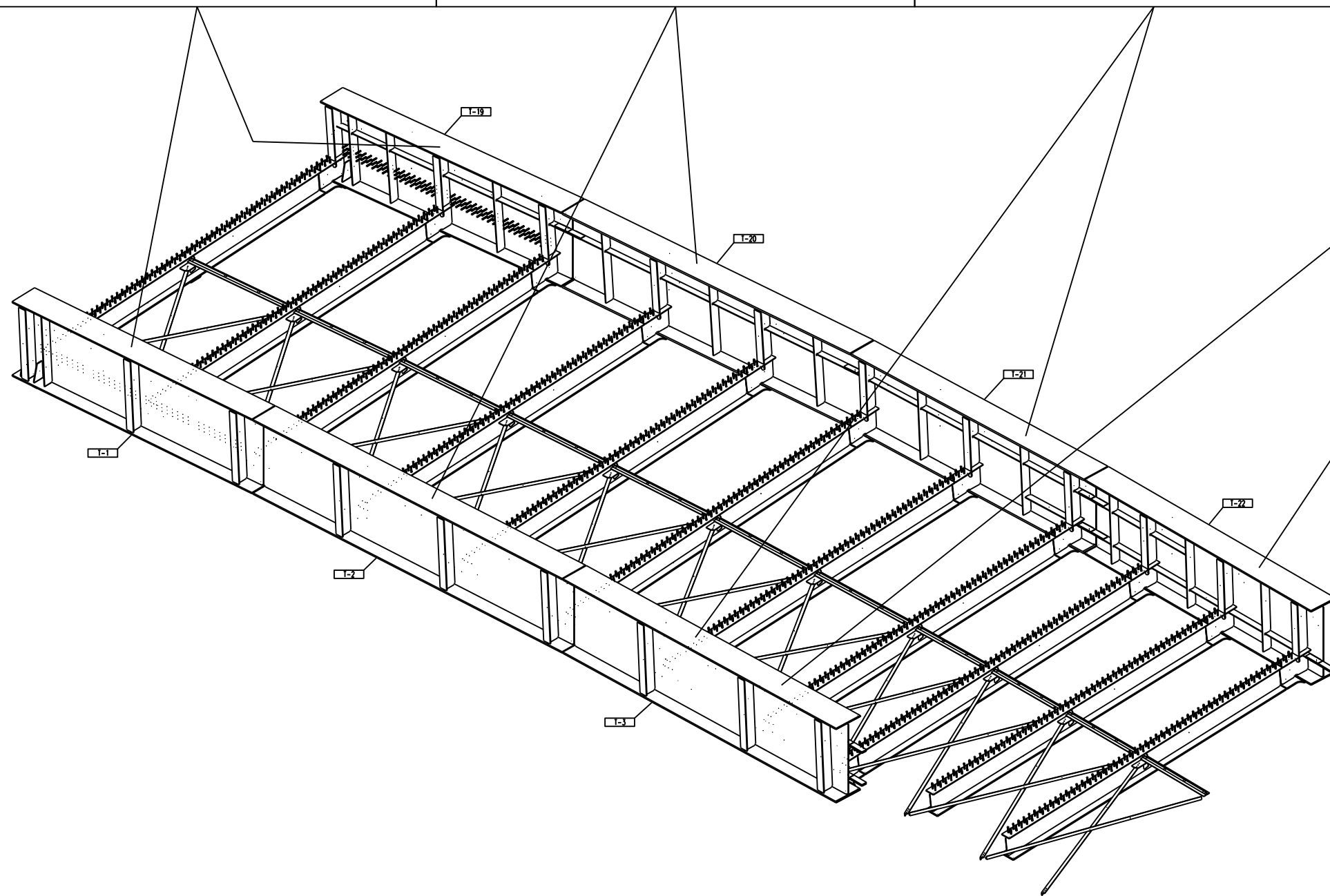
VISTA MISURE ESTERNE
