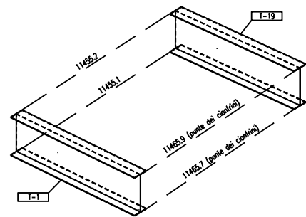
VISTA MISURE INTERNE
