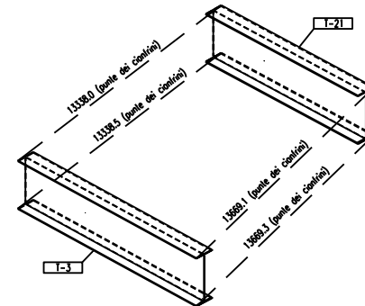
VISTA MISURE ESTERNE
