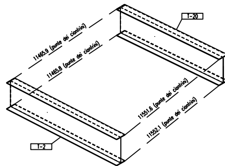
VISTA MISURE INTERNE
