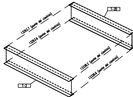
VISTA MISURE ESTERNE
