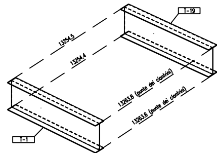
VISTA MISURE ESTERNE
