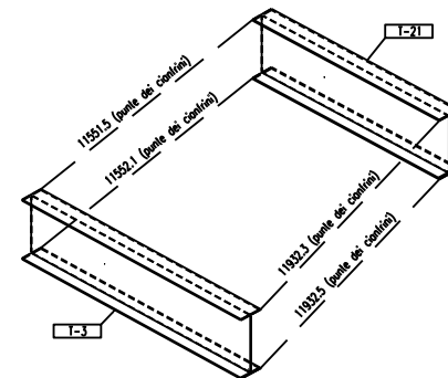
VISTA MISURE INTERNE
